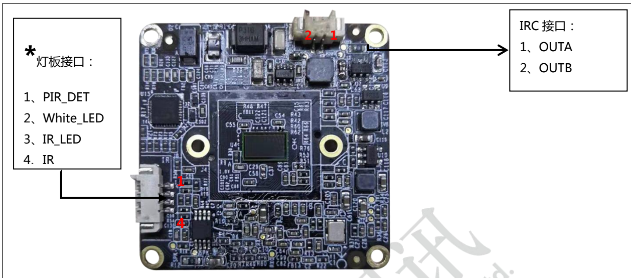
4-1主板正面图:
