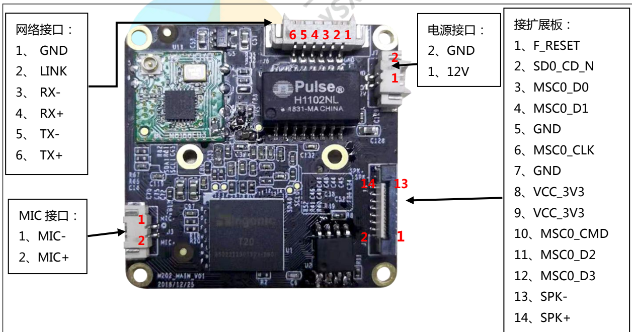
4-1 主板背面图：
