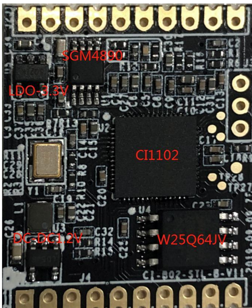
图 1 产品实物图
