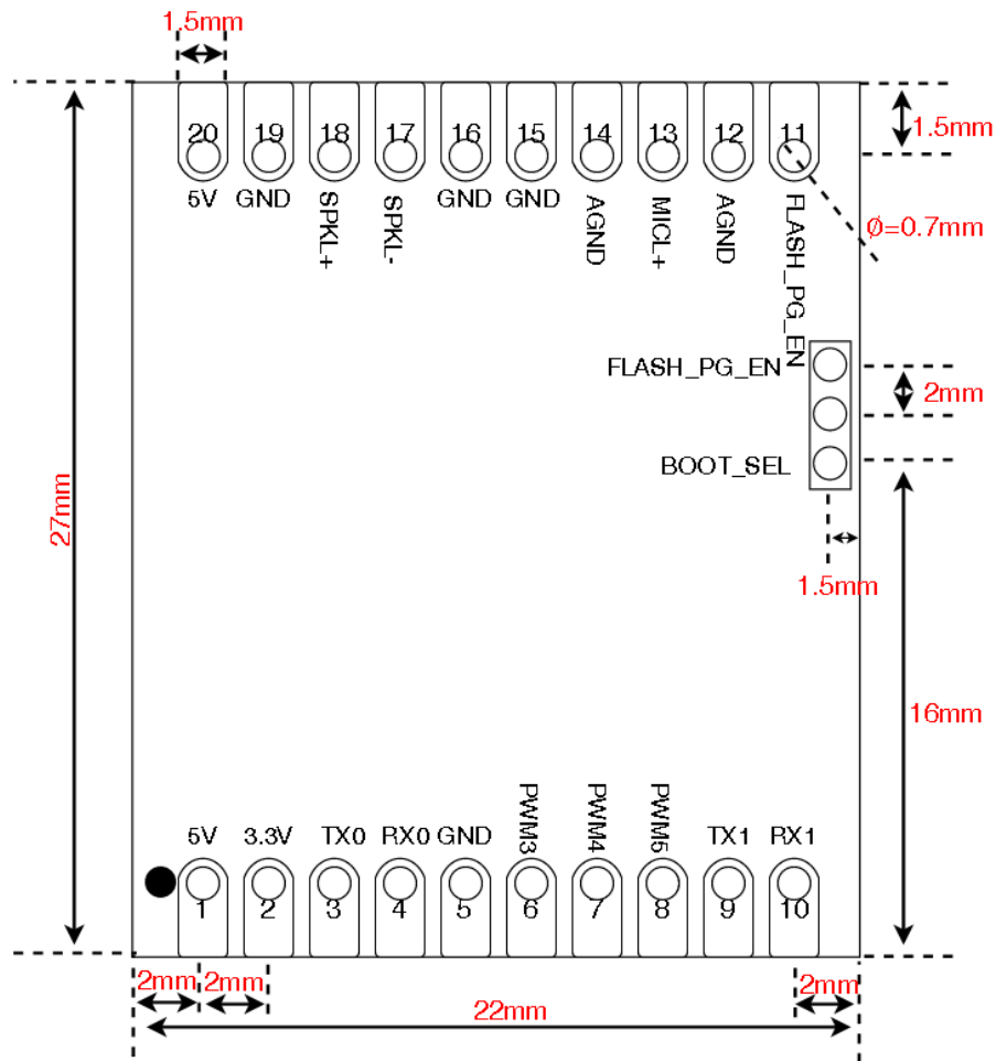
图 4 产品尺寸图
