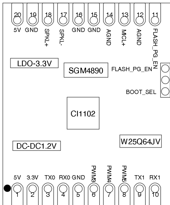
图 2 布局图
